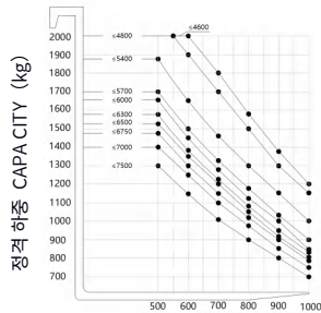
정격 부하 중심 거리 LOAD CENTER (mm)
