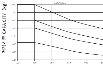
R20-L-부하 곡선CAPACITY CHART (mm) 고도 상승LIFT HEIGHT (mm)
