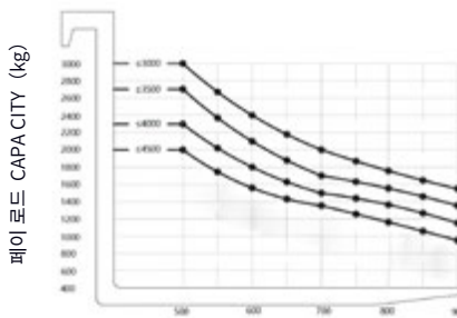
SE30-부하 곡선CAPACITY CHART (mm) 리프팅 높이LIFT HEIGHT (mm)
