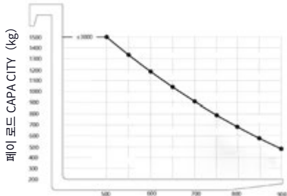
SE15-부하 곡선CAPACITY CHART (mm) 리프팅 높이LIFT HEIGHT (mm)
